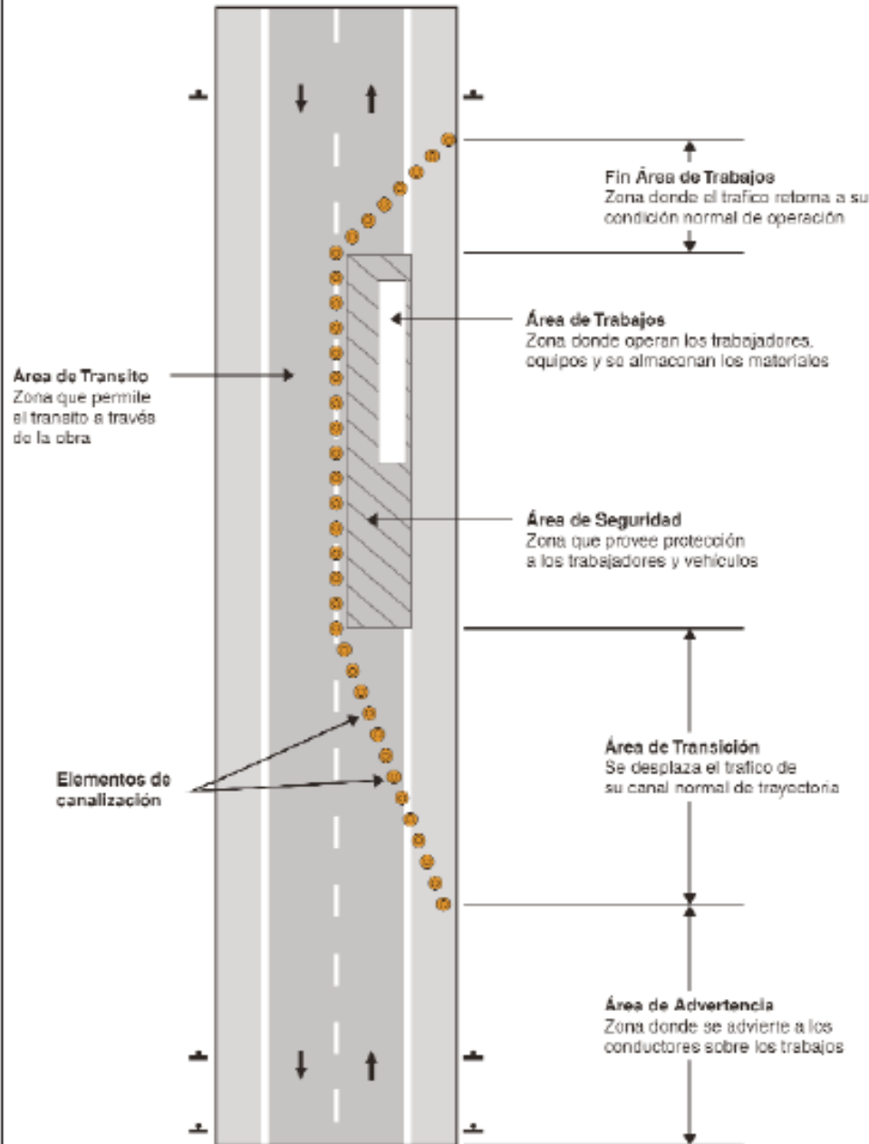
Figura 5.1. Zonas de trabajo en la vía
